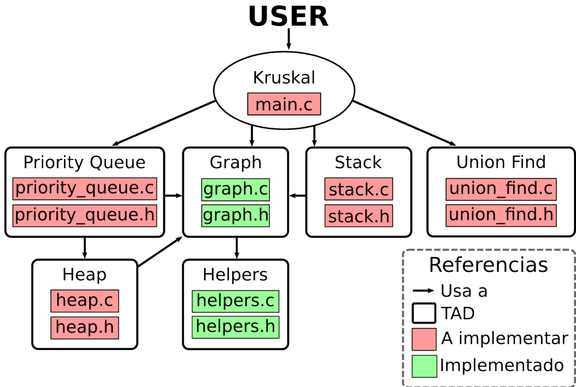
Figura 1: Diagrama de TADs
